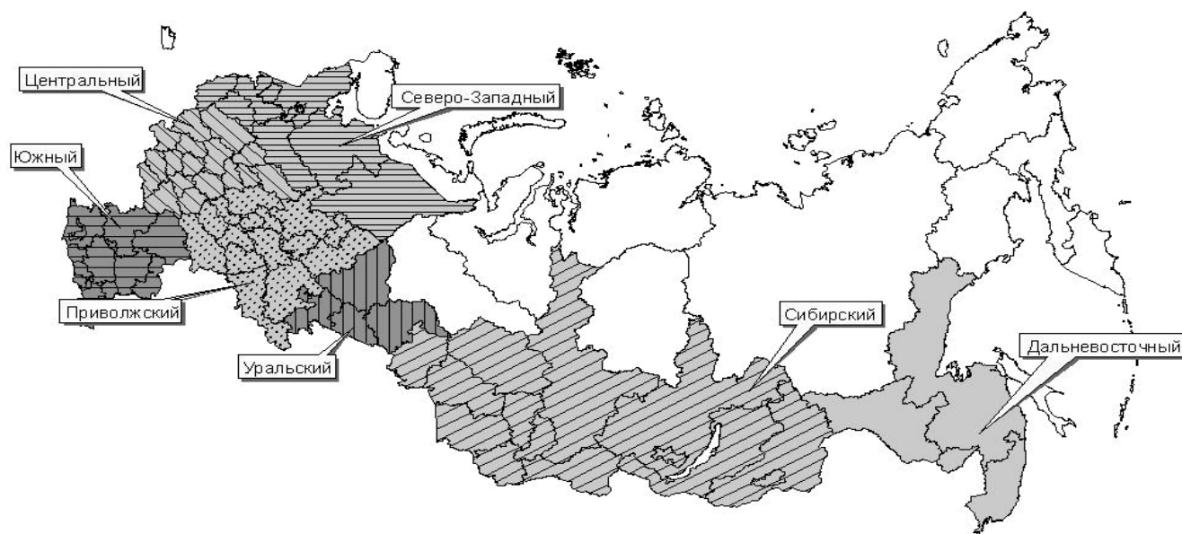
Рис. 2. Федеральные округа и области России, используемые для идентификации параметров модели АПКТ (включая тренды климатических факторов и тренд эффективности землепользования)
