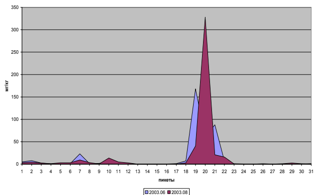
Рис. 4. Сезонная динамика НДМГ в горизонтах А и АВ бурых почв РП-25, к-1 а) в поверхностном (0-6 см) горизонте почв; б) в почво-грунтах (АВ 16-28 см)
