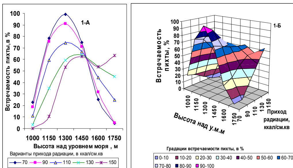
Рис. 1. Диаграммы встречаемости пихты сибирской в зависимости от высоты местности и инсолируемости склонов для Ивановского хребта северо-восточного лесорастительного района Рудного Алтая: 1-А – линии регрессии, 1-Б – поверхность регрессии в трехмерном пространстве.
