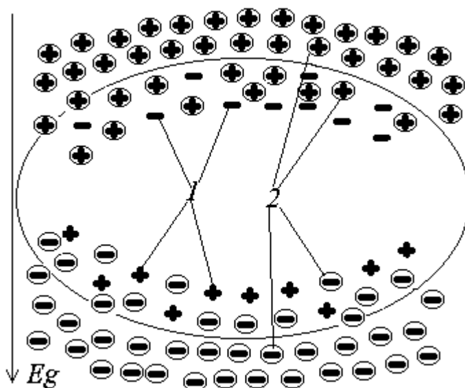
Рис. 2. Вакуумный эфиродомен в гравитационном поле Земли E_g (рассматривается физический вакуум вещества) с собственными связанными зарядами (1) МФВ накапливает атмосферные ионы (2).
