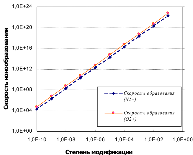
Рис. 1. Зависимость скорости ионообразования в теле ВЭД за счет фотоионизации.
