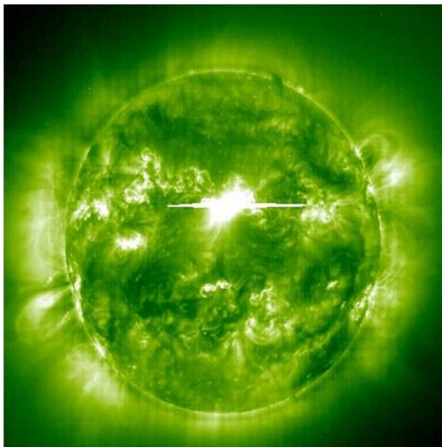
Рентгеновская вспышка 14 июля 2000 года. Снимок сделан в рентгеновском диапазоне на длине волны 195 ангстрем космическим зондом SOHO.
