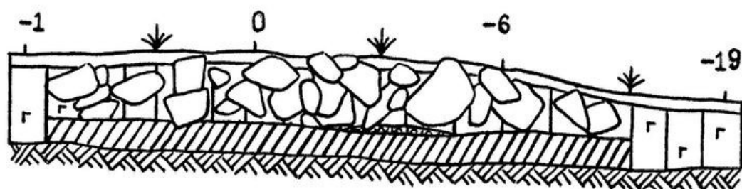
Рис. V. План и разрез оградки 3.
