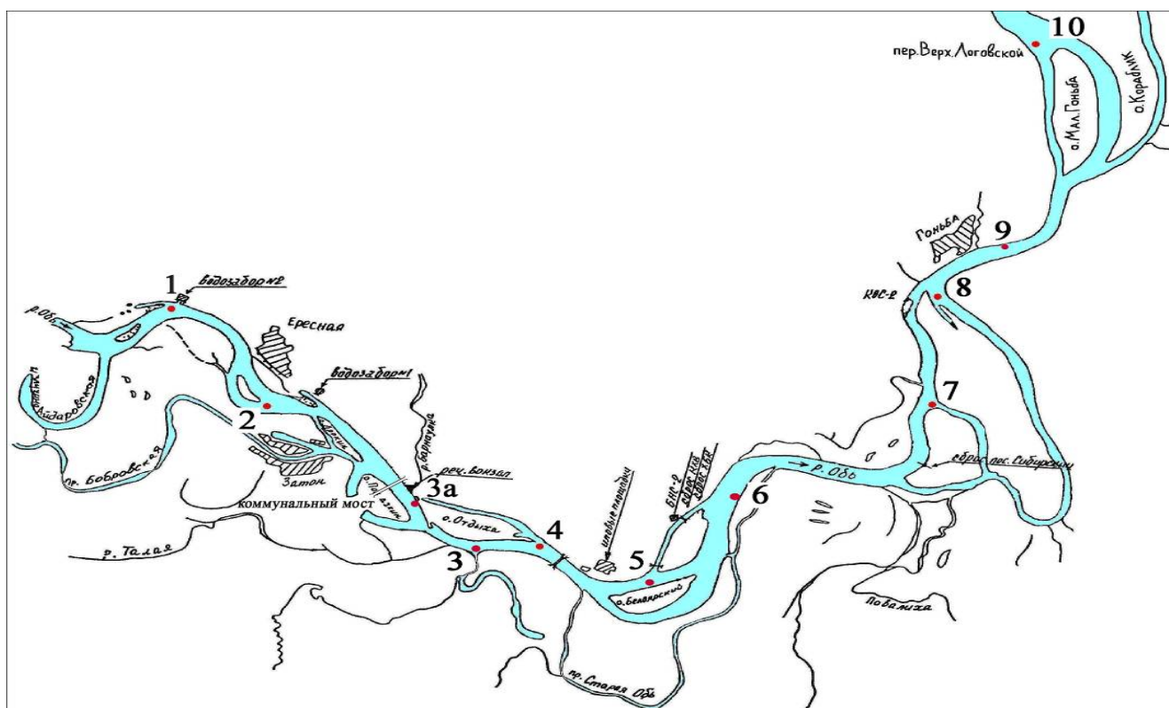
Рис. 1. Схема расположения створов на реке Оби в районе г. Барнаула
