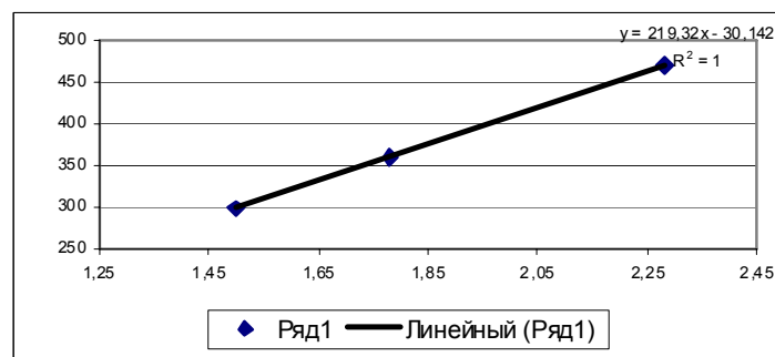
Рис. 3. Зависимость коэффициента концентрации (вертикальная ось) от площади ледника (горизонтальная ось, км²) [4]
