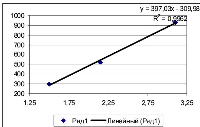
б) Рис. 4. Зависимость годового количества осадков (вертикальная ось, мм) от абсолютной высоты (горизонтальная ось, км) для южного склона Курайского (а) и северного склона Северо-Чуйского (б) хребтов.
