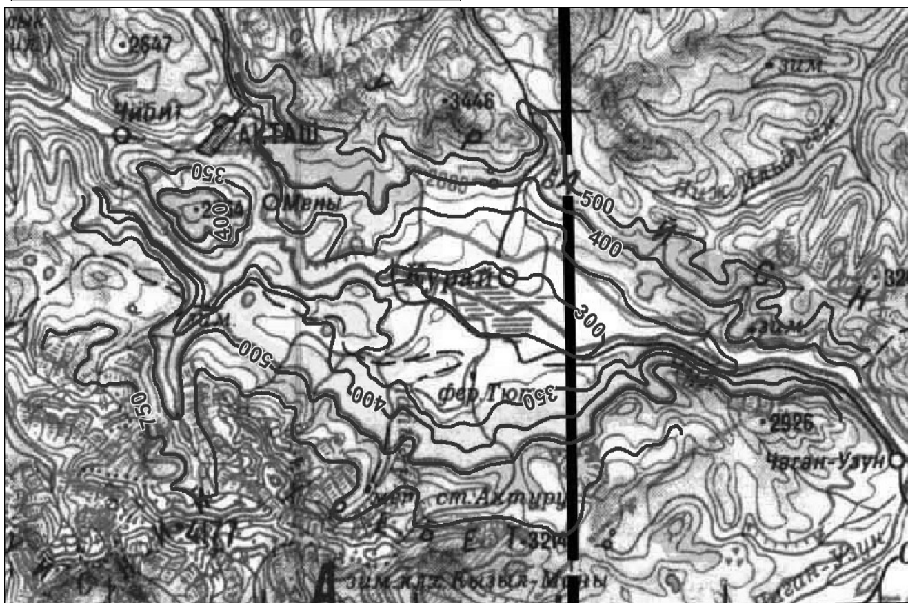
Рис. 5. Средние многолетние годовые осадки Курайской котловины
